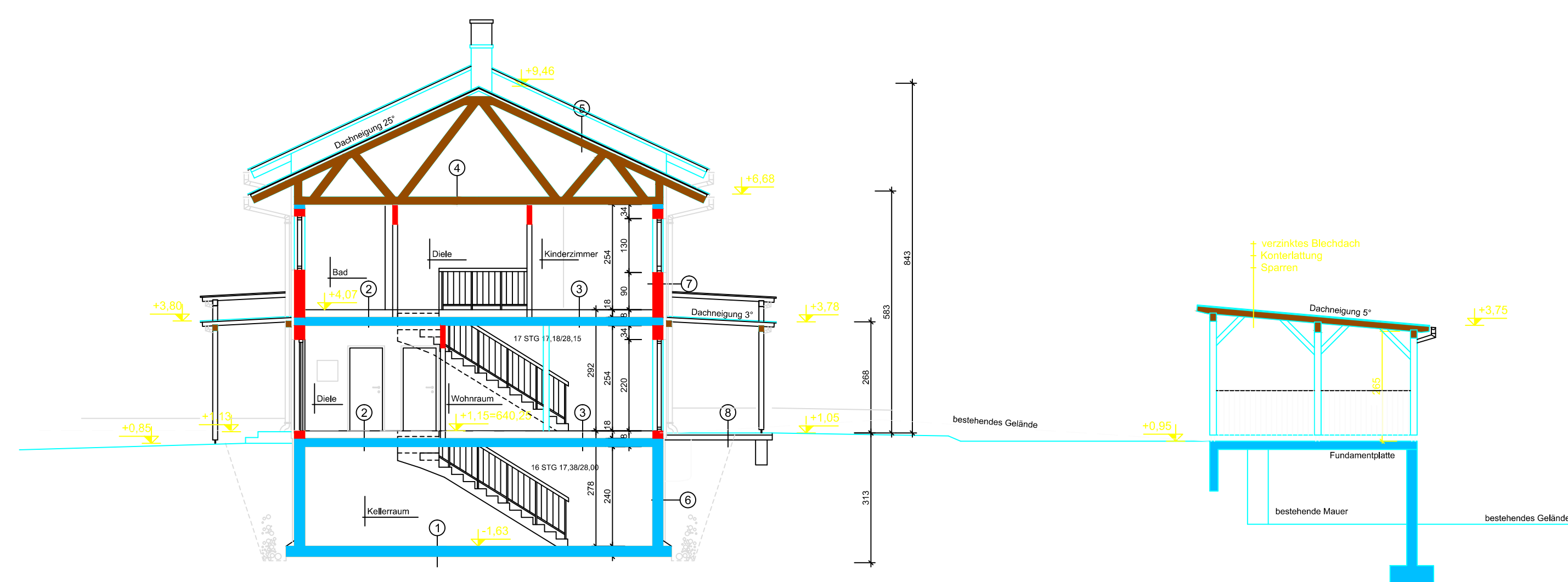
schnitt c-c maisonette 5
