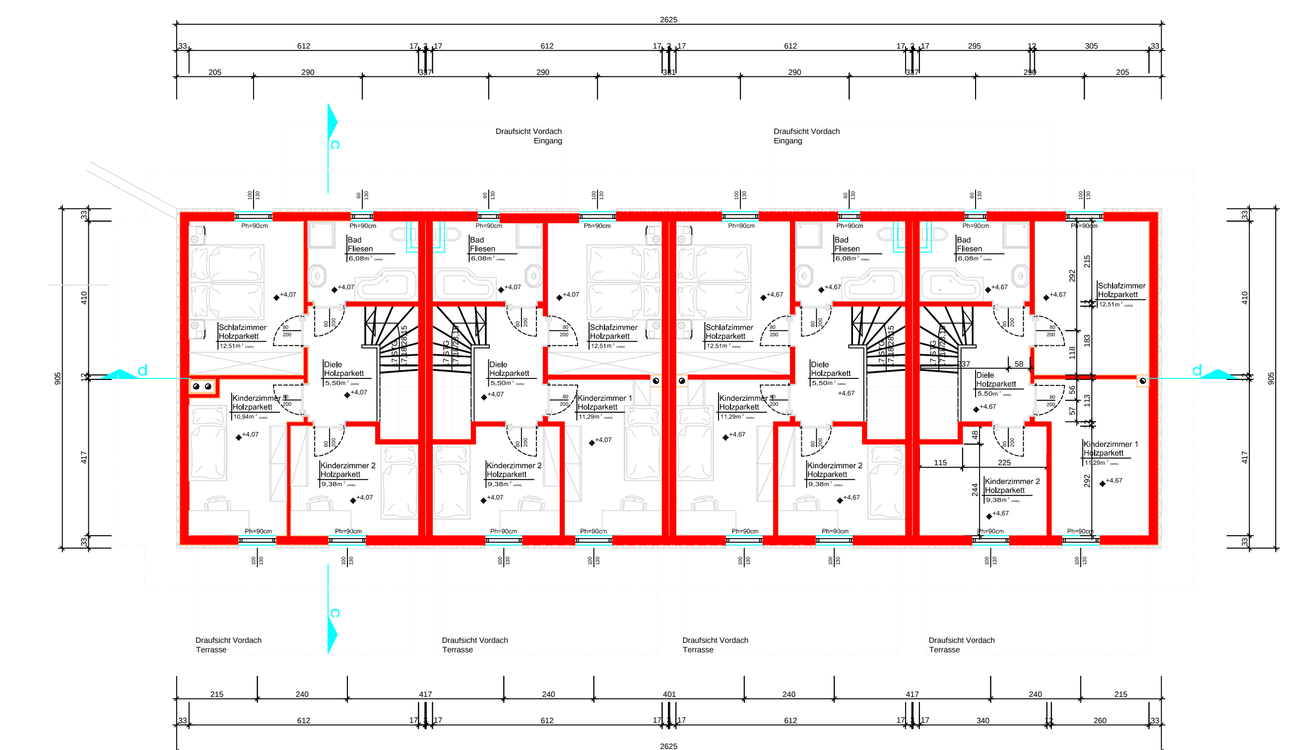
obergeschoß maisonette 5 bis 8
