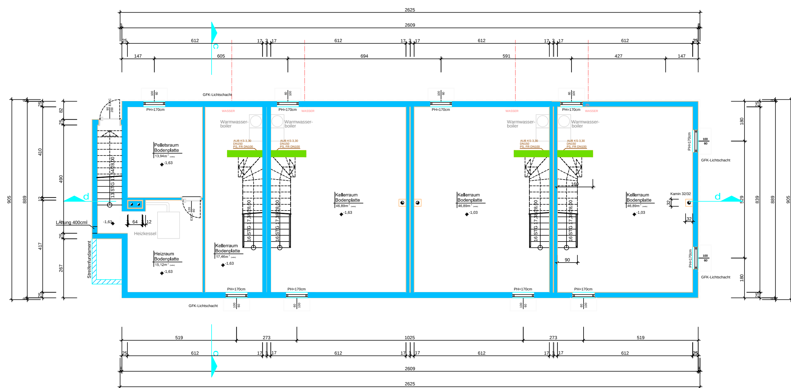
kellergeschoß maisonette 5 bis 8
