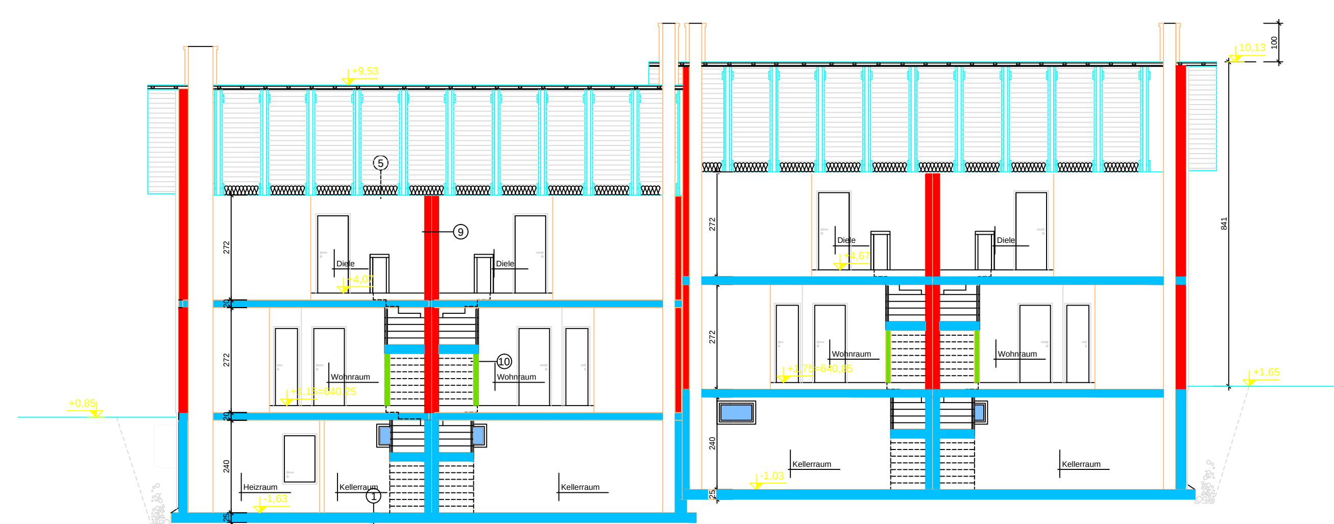
schnitt d-d maisonette 5 bis 8
